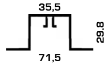
Einbauprofil für Glydea 595
